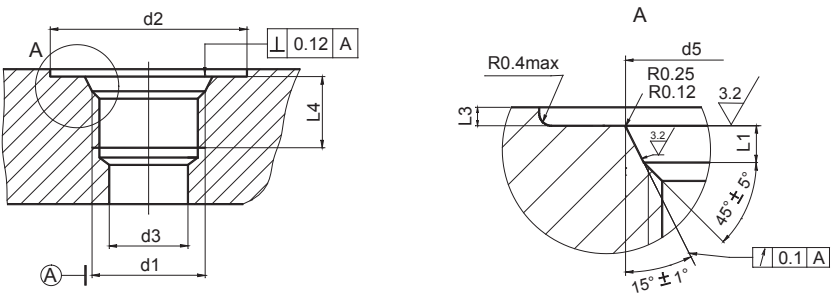
BS 5380油口
