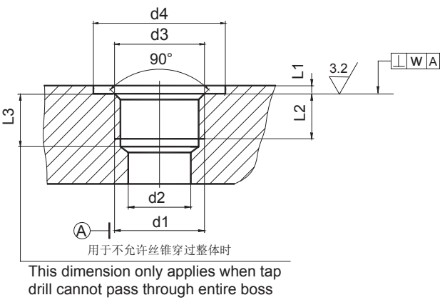
ISO 9974-1油口
