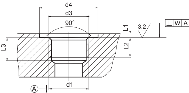
DIN 3852油口
