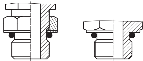
BS 5380柱端
